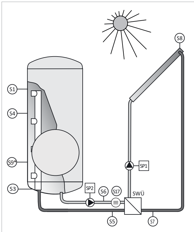
Abb. 8: Positionen der Sensoren SolvisBen * nur SolvisBen Solo
