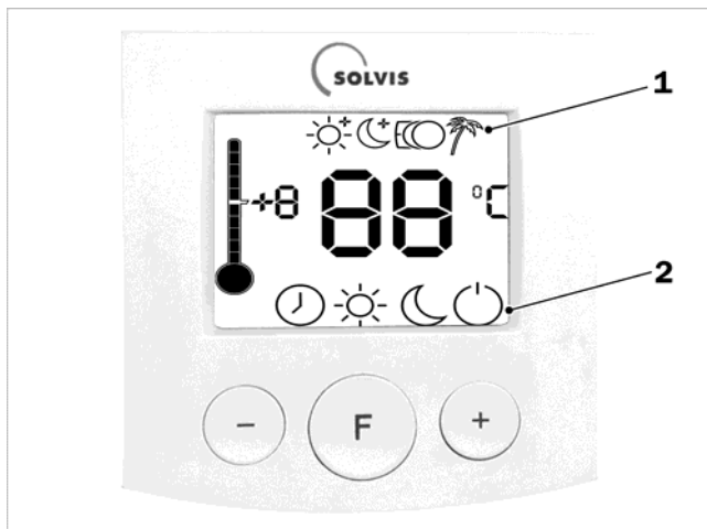
Abb. 2: Raumbedienelement BE-SC-2
