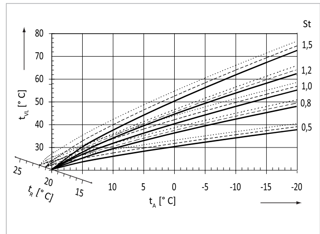
Abb. 11: Heizkurven bei diversen Raumsolltemperaturen
